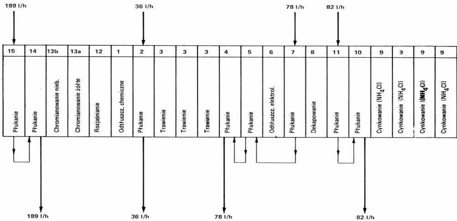
Galwanizernia duńska nr 3 - Schemat zmechanizowanej linii bębnowej do cynkowania
